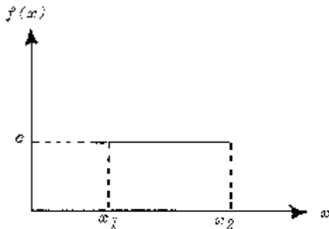
FIG. 2. Função de distribuição uniforme.
