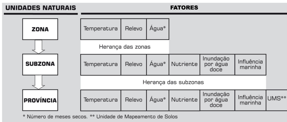
FIGURA 2 - Representação da hierarquia das Unidades Naturais com os fatores que participam de cada nível (FEITOZA, 2001a).
