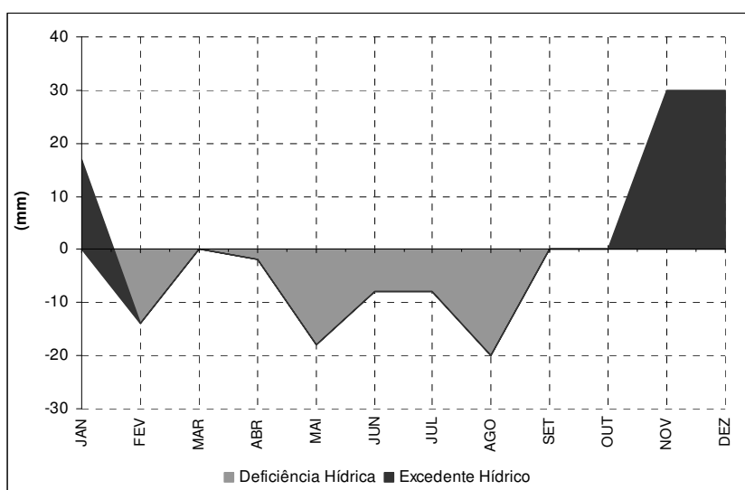
Figura 1. Gráfico do Extrato do Balanço Hídrico Climatológico do Município de São Mateus - ES, segundo THORNTHWAITE & MATHER (1955). Período: 1976-2006.
