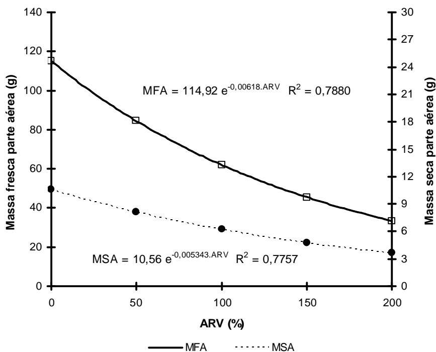
Figura 2 – Estimativa da massa fresca (MFA) e massa seca (MSA) da parte aérea das mudas do abacaxizeiro cv. Gold aos 180 dias após transplântio em função da adubação de referência para vasos (ARV).
