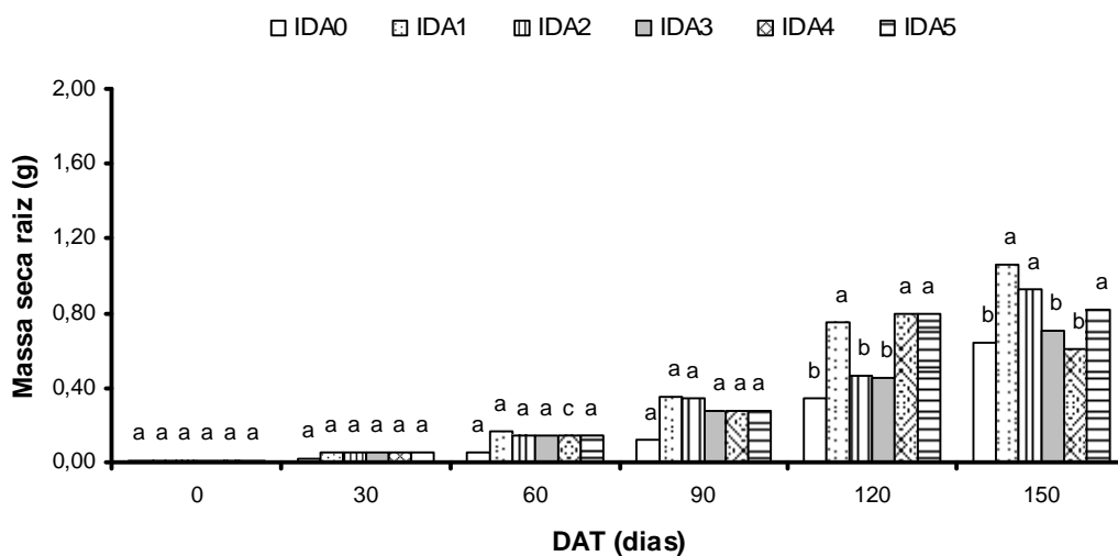
Figura 13 - Massa seca da raiz de mudas de abacaxizeiro cv. Gold em cada nível dos dias após transplante (DAT) para as idades de retirada da casa de vegetação (IDA).
