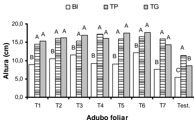
Figura 3 - Altura das mudas micropropagadas do abacaxizeiro cv. Gold aos 140 dias após o transplante para cada nível de adubo foliar em função dos níveis de recipientes: bandeja de isopor (BI), tubete pequeno (TP) e tubete grande (TG).
