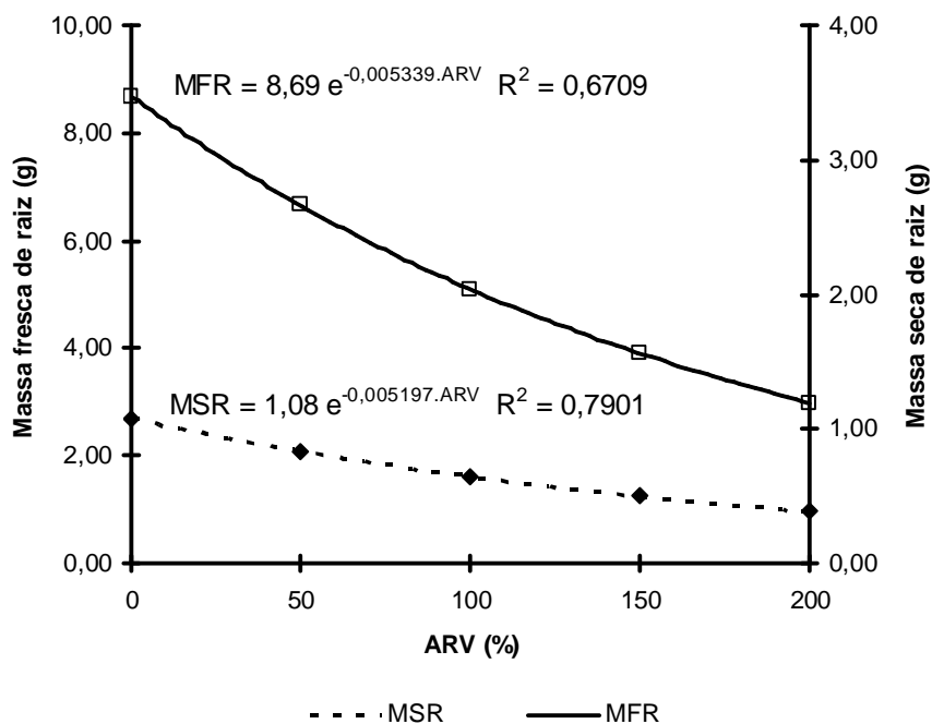
Figura 3 - Estimativa da massa fresca (MFR) e massa seca (MSR) da raiz das mudas do abacaxizeiro cv. Gold aos 180 dias após transplântio em função da adubação de referência para vasos (ARV).
