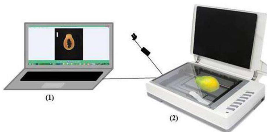
Figura 18 - Sistema de captura de imagens. (1) laptop e (2) modelo de scanner de mesa Optco Pro A32. (SANTA-CATARINA et al. , 2018).
