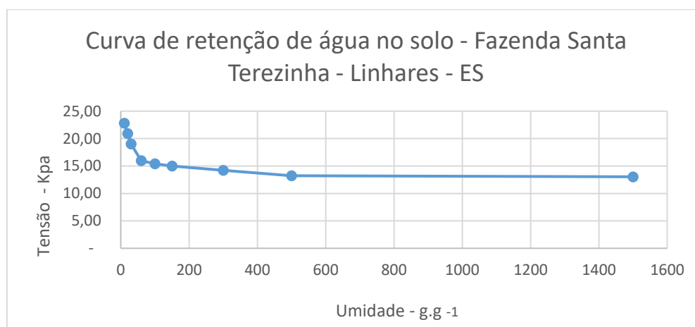
Figura 6 - Curva padrão de umidade do solo
