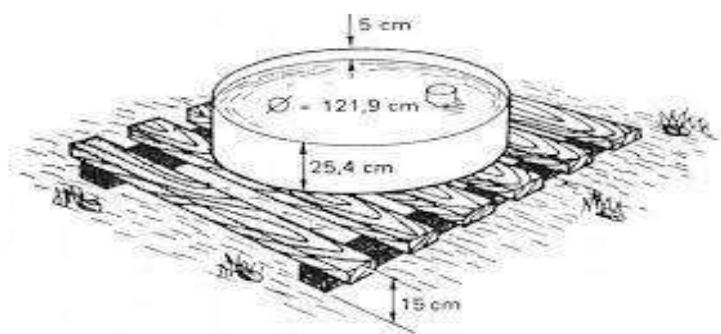
Figura 2 - Dimensões do Tanque Classe A.
