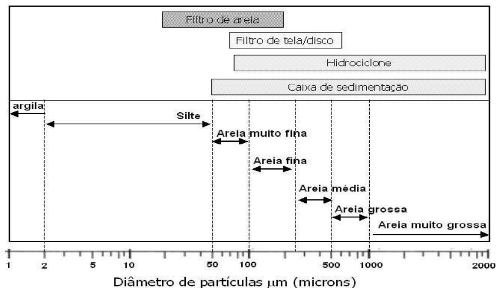
Figura 10 - Recomendação para uso de filtros [Fonte: Pizzaro Cabello (1990; 1996)].
